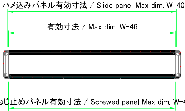
A-A ( 1 : 10 )
