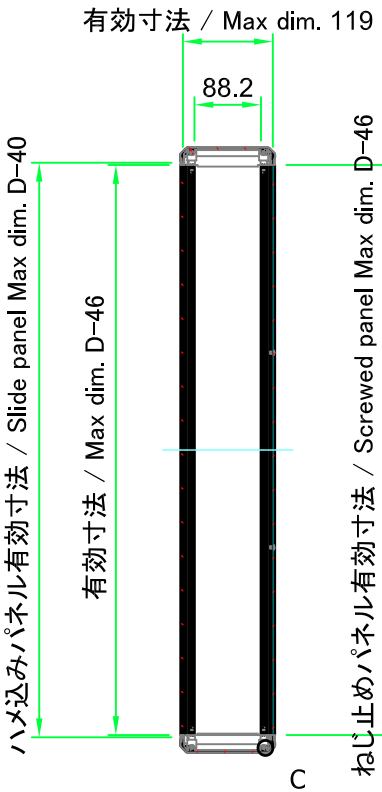
B-B ( 1 : 10 )
